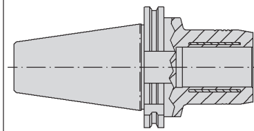
SK-Aufnahme
