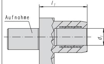
VDI-Aufnahme
