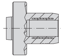
Flansch mit Aussenkegel
