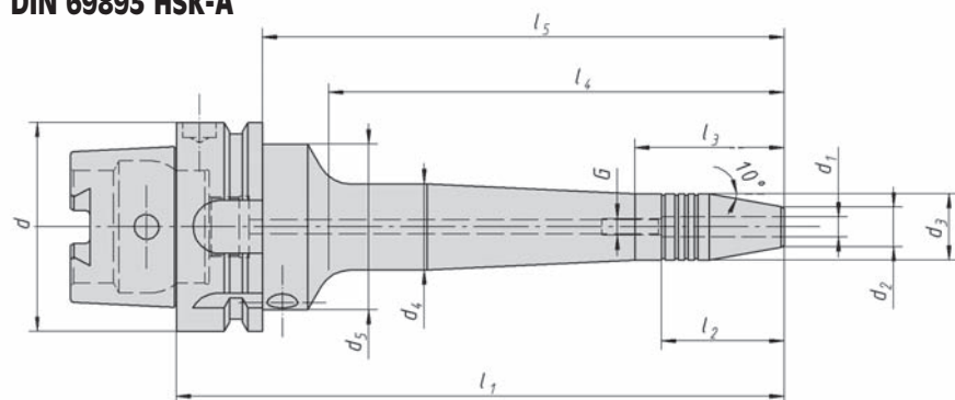
DIN 69893 HSK-A
