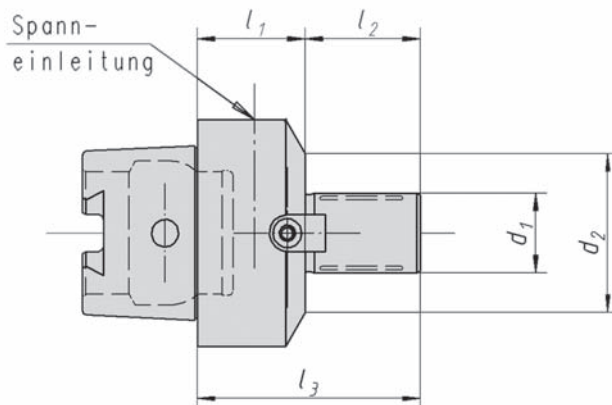
HSK-C63 DIN 69893
