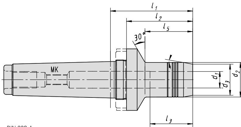
DIN 228-A
